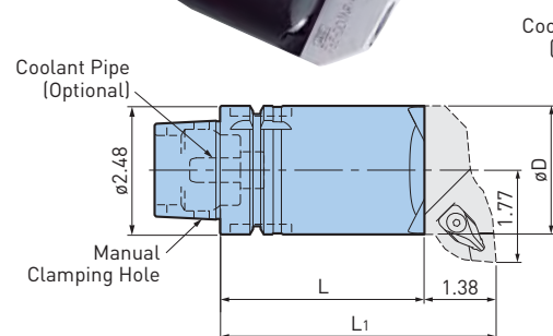
Fig. 1 (HSK-T63)
