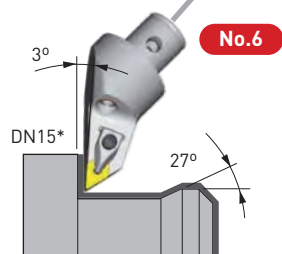
S50-DDJNR-33075-15 -DDJNL-33075-15
