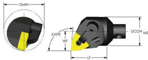
NEGATIVE TRIGON (KAPR: 95°)
