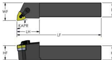
NEGATIVE TRIGON (KAPR: 95°)
