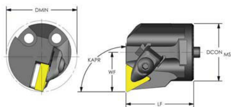
PULLBACK CLAMP NEGATIVE TRIANGLE (KAPR: 90°)
