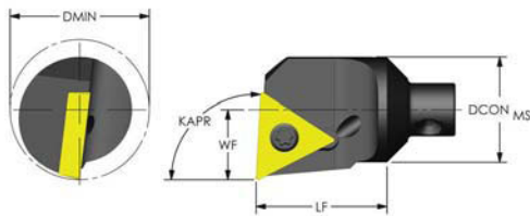
POSITIVE TRIANGLE (KAPR: 93°)
