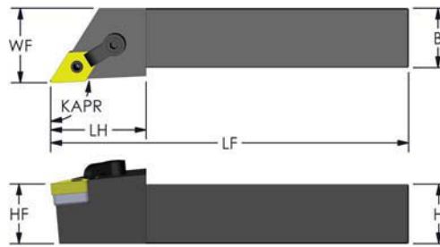
NEGATIVE 55° DIAMOND (KAPR: 93°)
