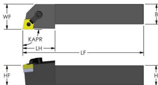
NEGATIVE 80° DIAMOND (KAPR: 90°)
