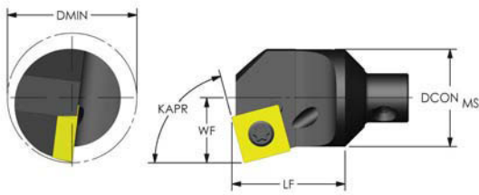
POSITIVE SQUARE (KAPR: 75°)
